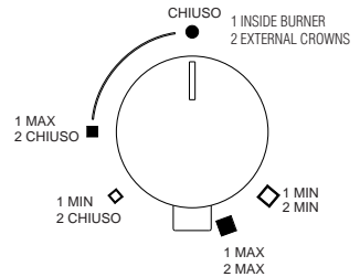
Fig. 13: burner knob dual (GIOTTO/VULCANO)
